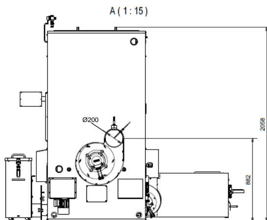
UTSD 240 CH vL (120-260 kW)
