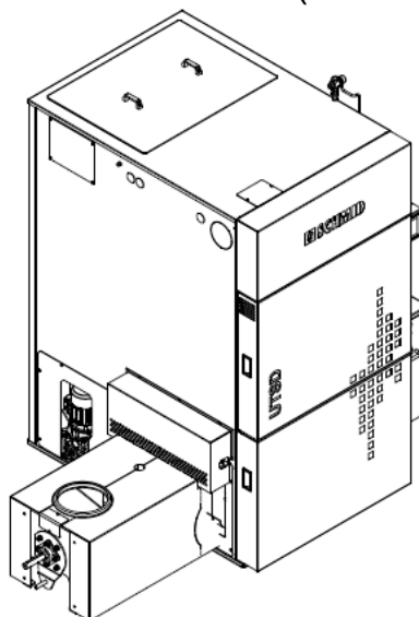
UTSD 240 CH vL (120-260 kW)
